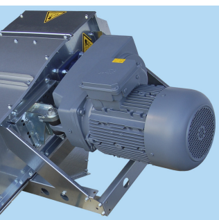
Direktmonterad tappväxelmotor med stagarm.
